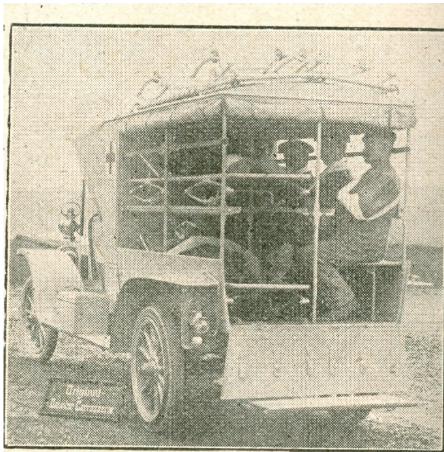
Abb. 8. Mercedes-Militärsanitätsautomobil.
